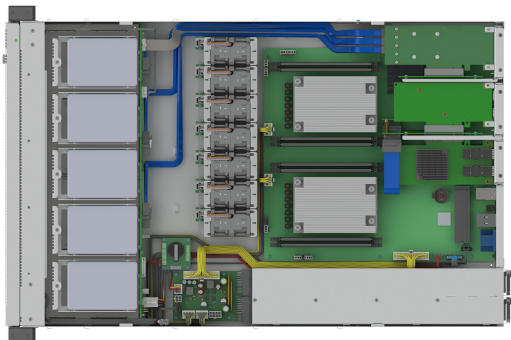
Сервер "НОРСИ-ДРАКОН" 4LFF / Вид сверху
