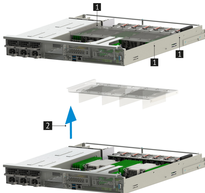
Рис. 24. Извлечение воздушного кожуха
