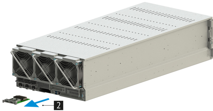
Рис. 53. Извлечение карты OCP 3.0 PCIe x16
