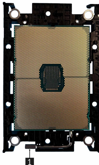
Рис. 39. Снятие процессора с радиатора
