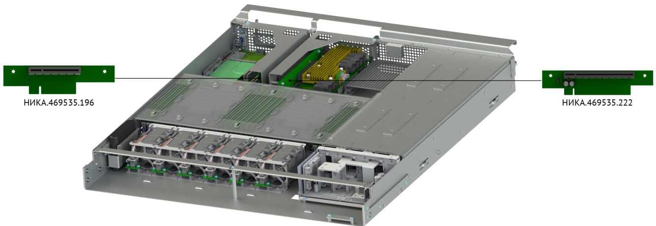
Рис. 11. Расположение PCIe-райзеров в модуле НИКА.467239.008 сервера
