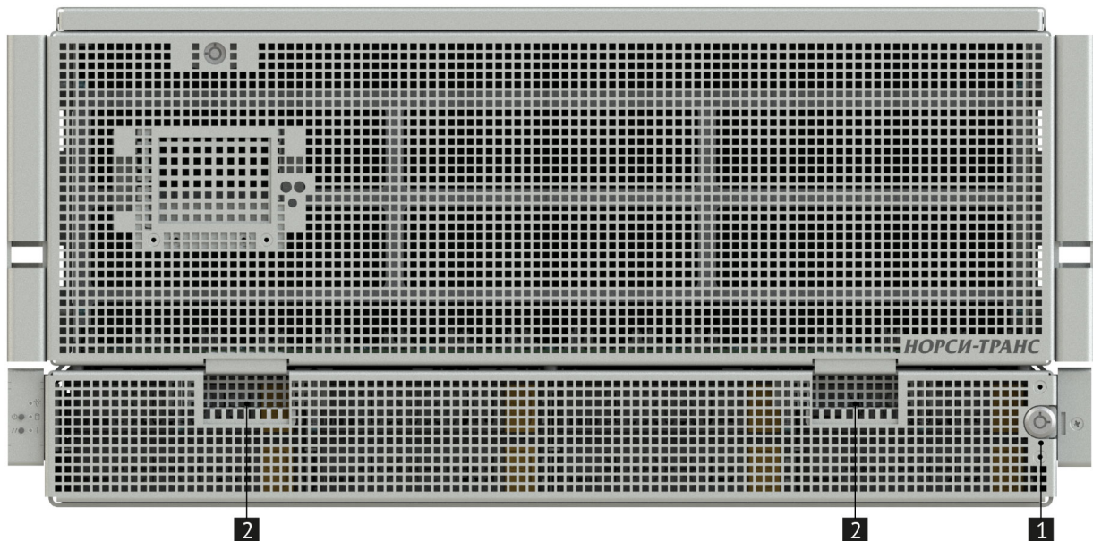
Рис. 16. Открытие передней панели ключом
